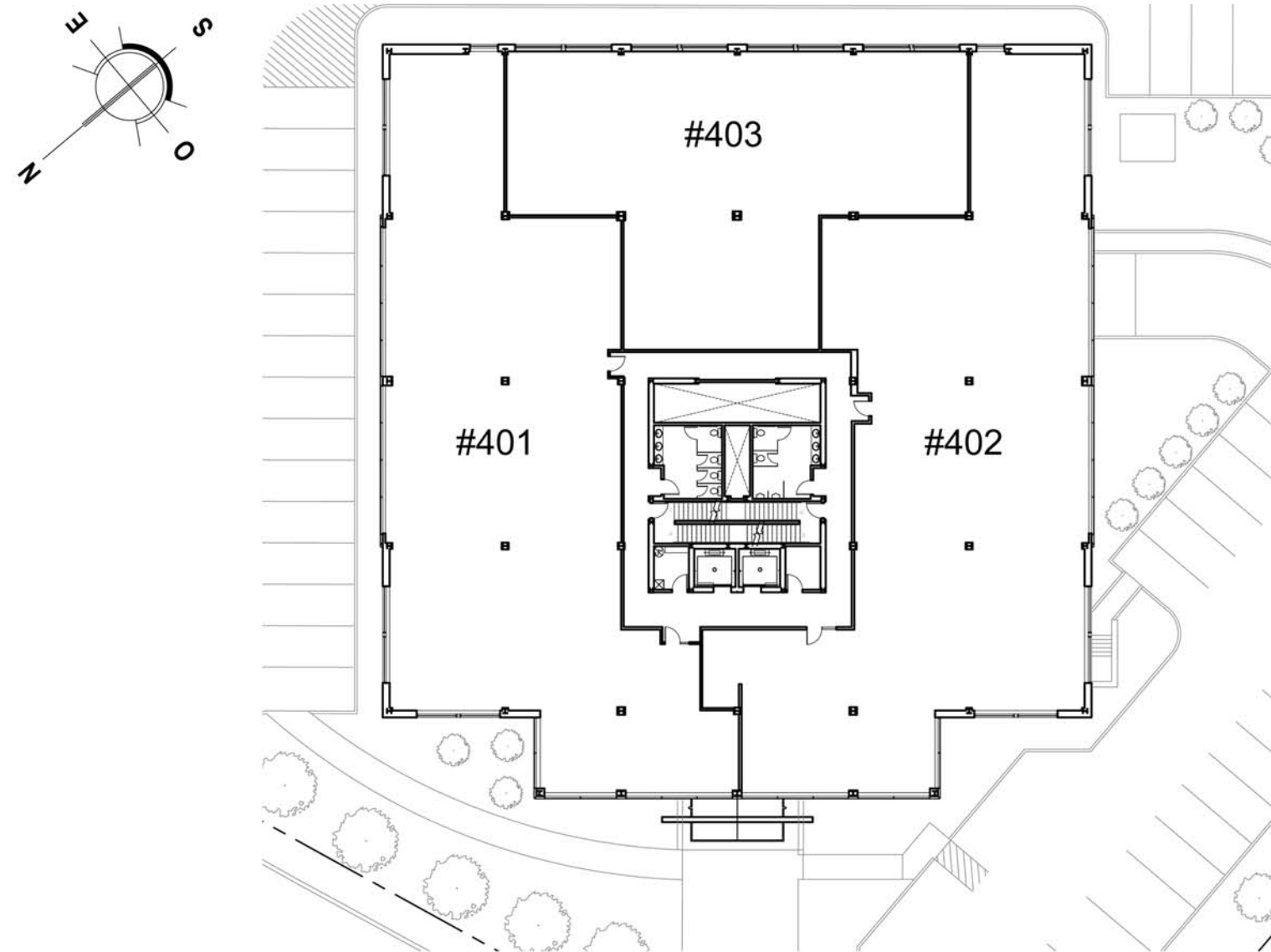
4ième ÉTAGE
